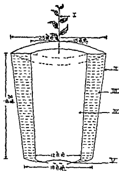
चित्र 10. परिवर्धित गमले का अनुदध्य काट। I. पौधा, II. रंग से पुती हुई सतह, III. पानी, IV. मिट्टी और V. खुला हुआ भाग।
