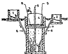
चित्र 9. गोबर-गैस प्लान्ट। (1) गोबर भरने का कक्ष (2) पाचित स्लरी के लिये कक्ष (3) गैस की निकासी का मार्ग (4) टंकी (5) टंकी को सीधा रखने के लिये पाइप (6) स्लरी के निकासी के लिये पाइप (7) दीवार (8) गैस और (9) स्लरी।
